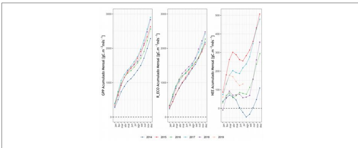
Figura 4.13 – Série mensal de GPP, R_{ECO} e NEE, acumulado, para todo período analisado.
