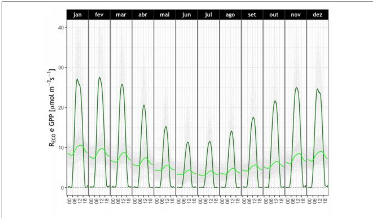
Figura 4.15 – Evolução mensal média do ciclo diário de GPP (linha verde forte) e R_{ECO} (linha verde claro).
