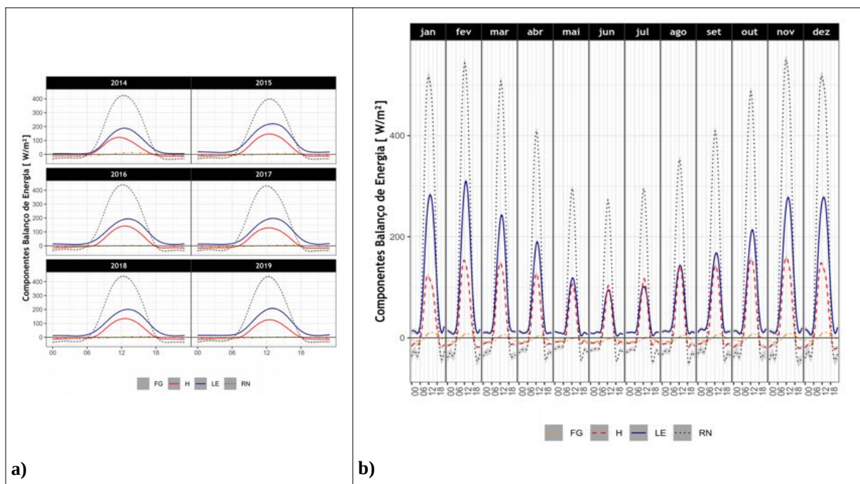
Figura 4.5 - Ciclo diário médio das componentes energéticas, são elas: R_N (Radiação líquida), F_G (Fluxo de Calor no Solo), H (Fluxo de Calor Sensível) e LE (Fluxo de calor Latente), a) anual e b) mensal.
